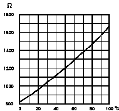
Framledningsgivare T1
